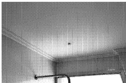
FOTO 14: APTO Nº 1101 – INFILTRAÇÃO NO FORRO DO WC
