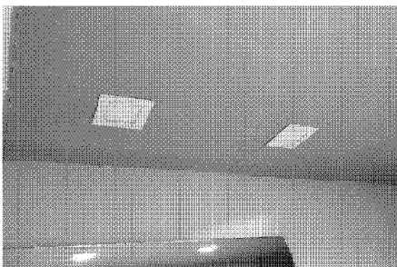
FOTO 62: SUÍTE 321 - INFILTRAÇÃO NO FORRO DO WC
