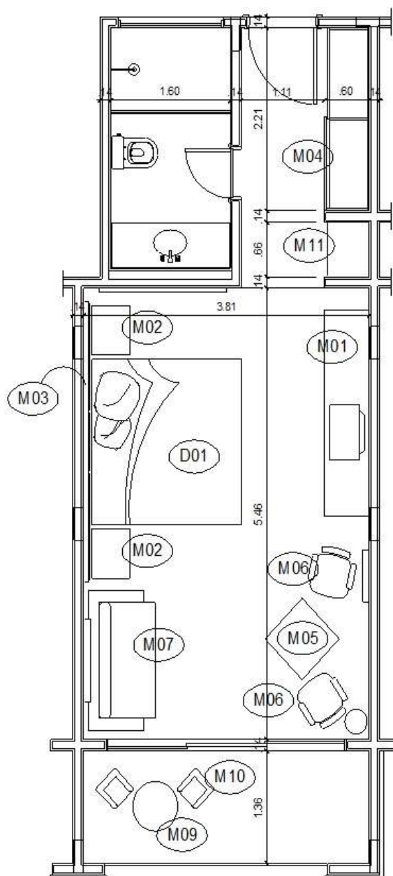
2 PLANTA BAIXA - CASAL ESCALA: 1/50
