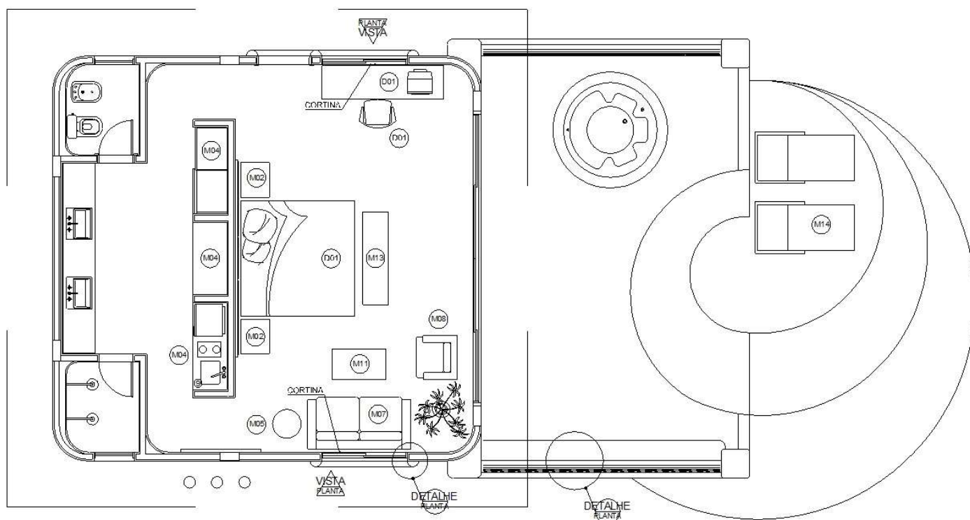
1 PLANTA BAIXA ESCALA: 1/50
