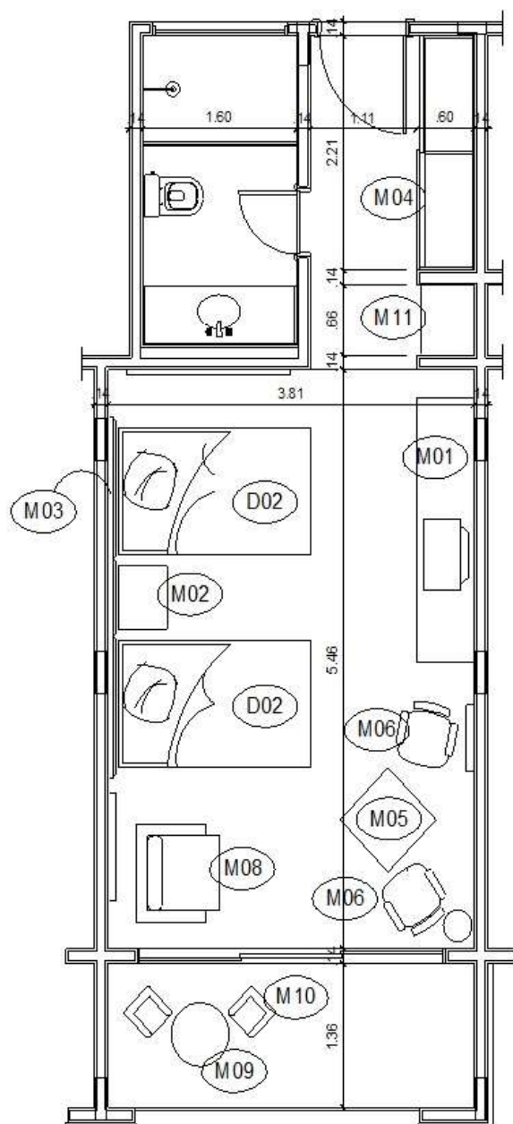
1 PLANTA BAIXA - SOLTEIRO ESCALA: 1/50
