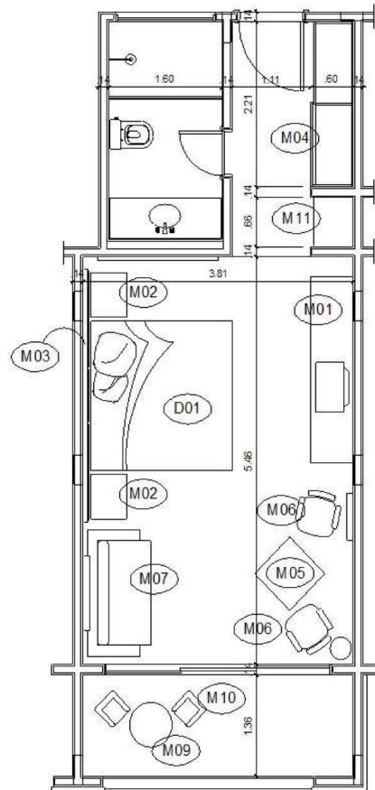
2 PLANTA BAIXA - CASAL ESCALA: 1/50
