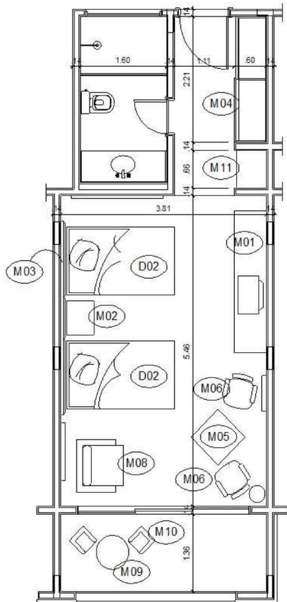
1 PLANTA BAIXA - SOLTEIRO ESCALA: 1/50
