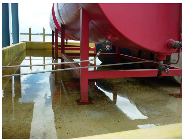
caixa coletora do tanque de combustível do motor-bomba de combate a incêndio
