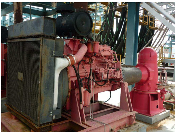
Motor bomba de combate de incêndio
