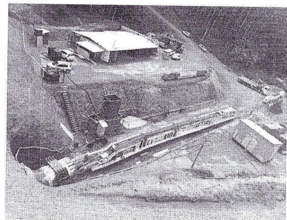
Vista geral da máquina
