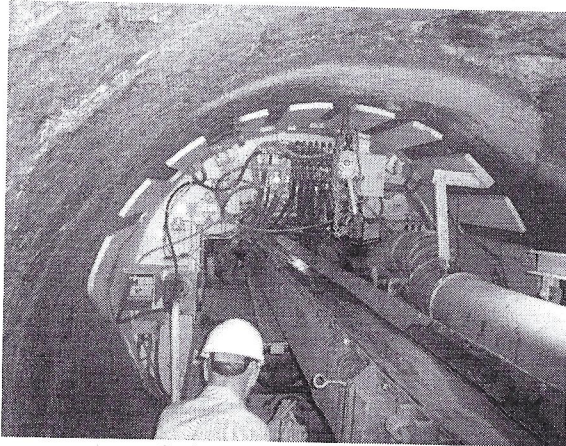
Cabeçote de corte
