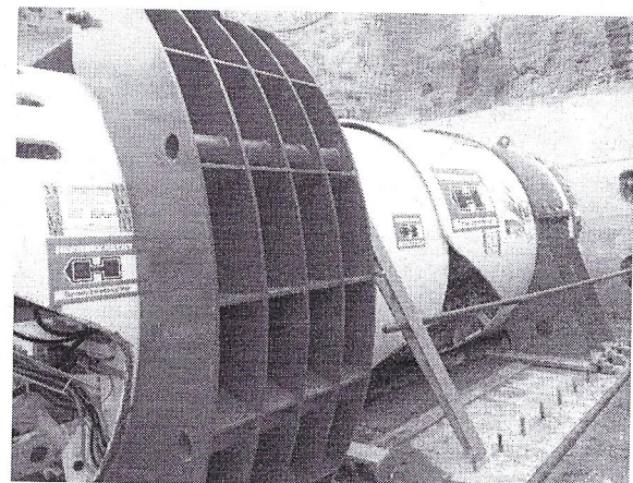
Frente da máquina
